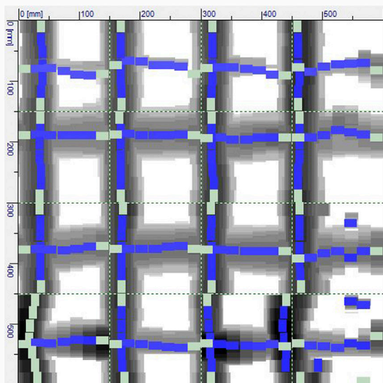
Determinación de diámetros, recubrimiento y espaciamiento
