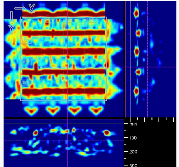
Localización de cavidades (placa alveolar)
