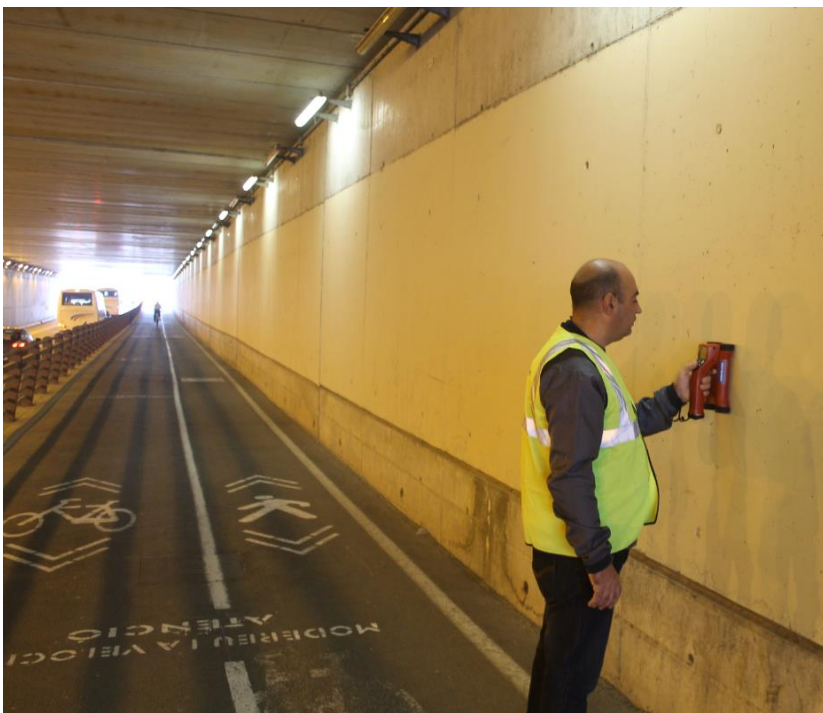
Detección / verificación de armados
