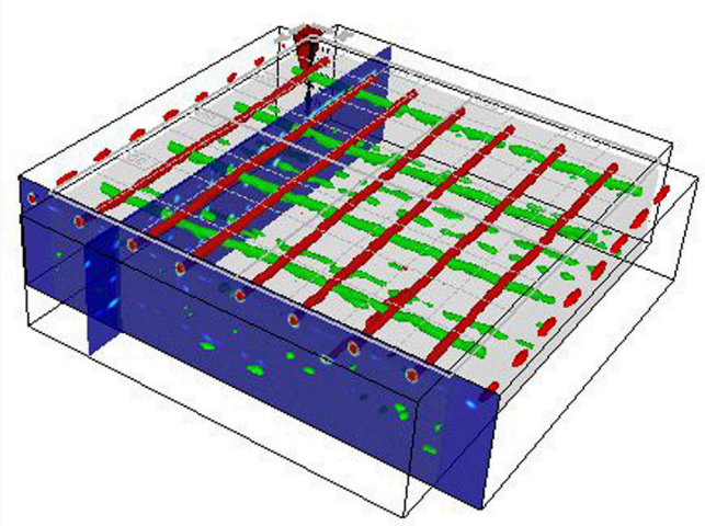
Vista 3D del armado del hormigón
