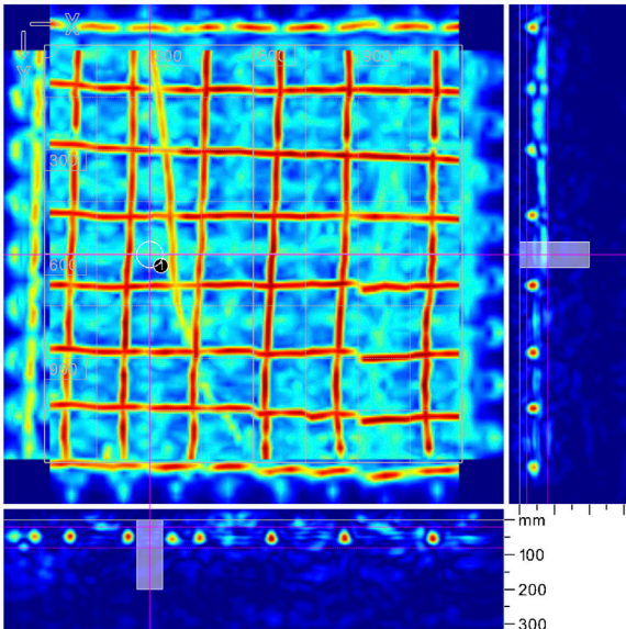
Vista 2D del armado, taladros y cable
