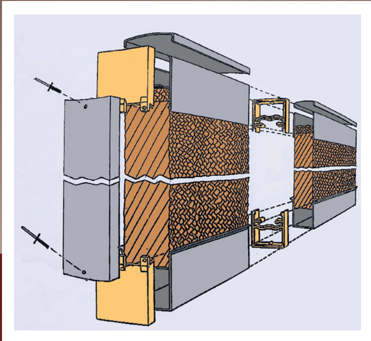
Sistema de refrigeración con paneles evaporativos
